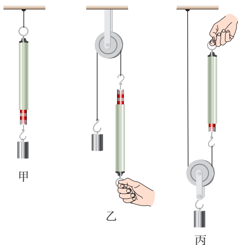
图12.3-4 研究定滑轮和动滑轮的特点
