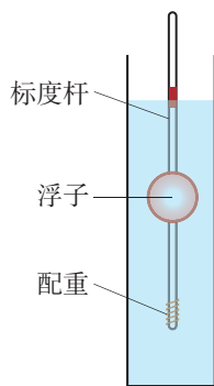
图10.4-4 微型密度计的构造
