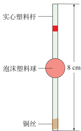
图10.4-5 一种微型密度计
