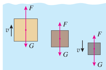
甲上浮 乙悬浮 丙下沉
