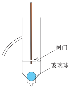
图9.4-6 简易活塞式抽水机结构图
