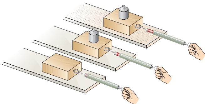
图8.3-4 探究滑动摩擦力
