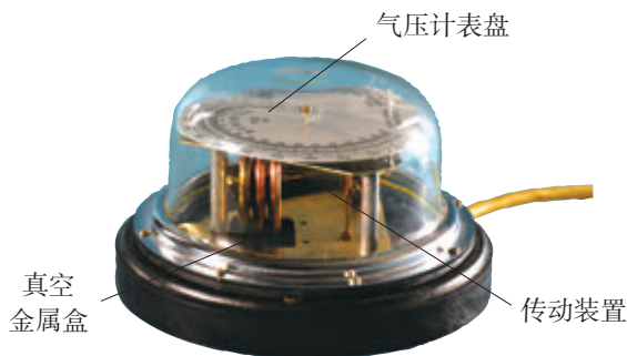
图9.3-4 无液气压计
