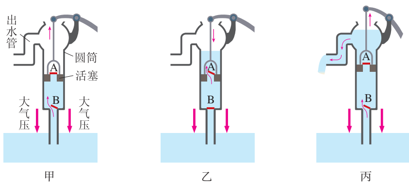
图 9.4-2 活塞式抽水机工作原理示意图
