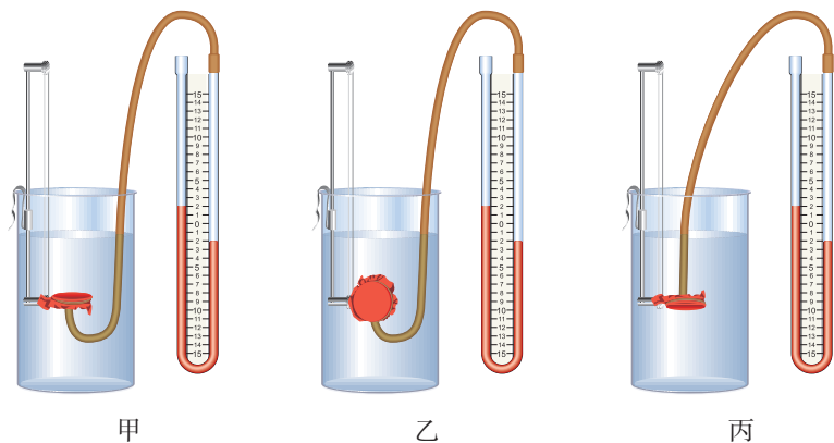
图9.2-3 同一深度各个方向的压强
