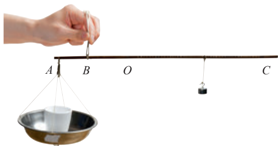
图12.2-2 自制杆秤
