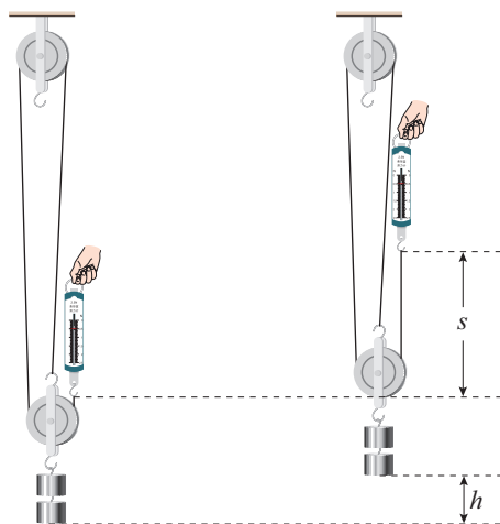
图12.4-2 测量滑轮组的机械效率
