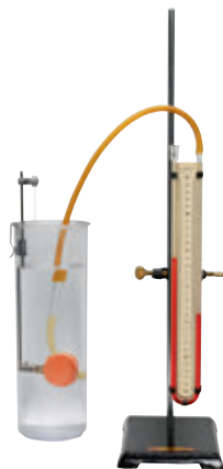
图9.2-2 测量液体压强
