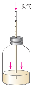
图9.3-5 自制气压计
