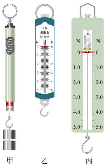
图7.2-2 弹簧测力计
