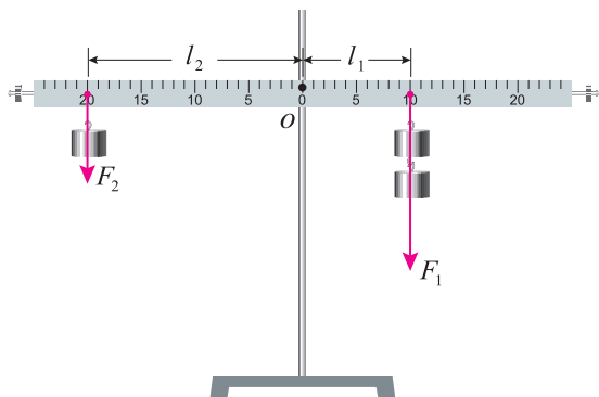
图12.1-3 探究杠杆的平衡条件
