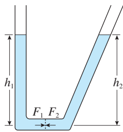
图9.2-6 连通器中液面的高度相同
