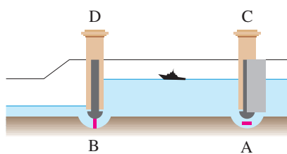
图9.2-8 三峡船闸
