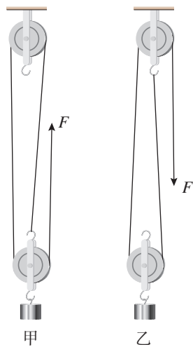
图12.3-5 定滑轮和动滑轮可以组成滑轮组
