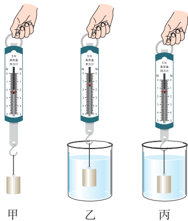
图10.1-3 测量铝块所受的浮力
