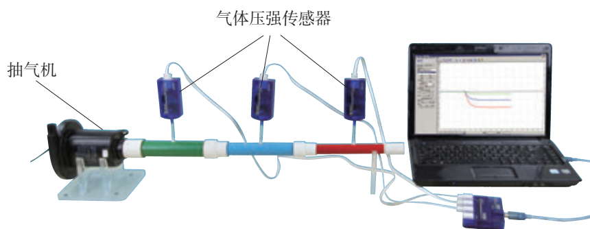
图9.5-4 研究气体压强与流速的关系
