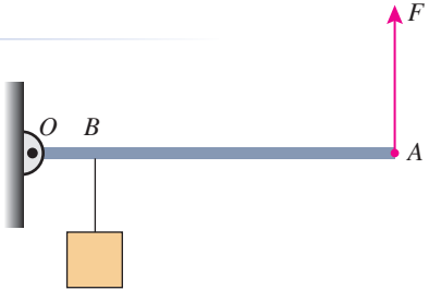
图12.1-4 一种杠杆
