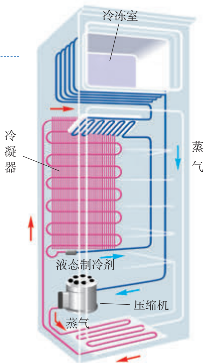
图3.3-7 一种电冰箱的原理图
