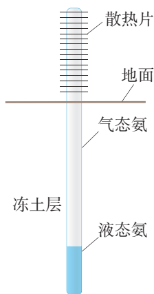
图3.3-9 热棒示意图
