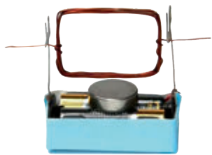
图2 转动的线圈
