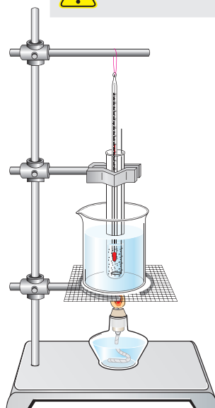
图 3.2-2 观察熔化现象的实验装置
