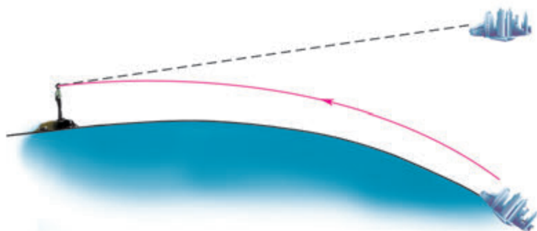
图4.4-6 海市蜃楼的成因
