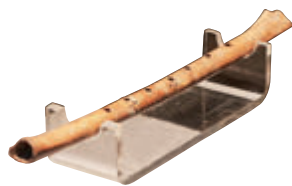
图2.2-6 贾湖骨笛
