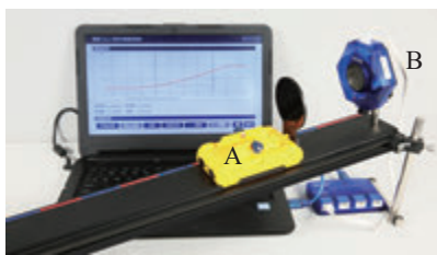
图1.4-3 利用传感器测量物体运动的速度
