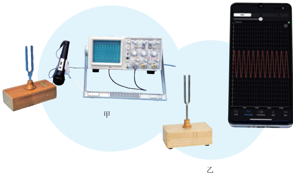
图2.2-3 声音的波形
