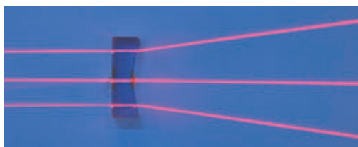
图5.1-6 凹透镜使光发散
