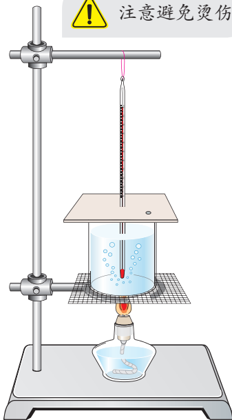
图 3.3-2 观察水沸腾的实验装置
