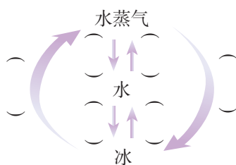
图3.4-3 水的三态联系
