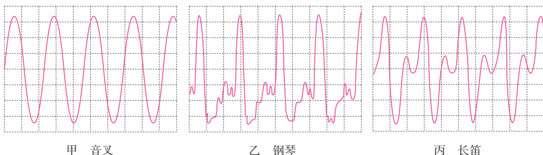
图2.2-5 声音的波形
