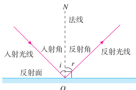
图4.2-5 光的反射
