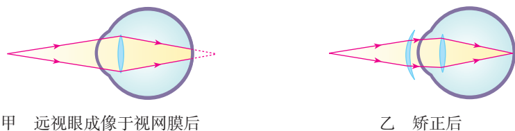
图5.4-4 远视眼及其矫正
