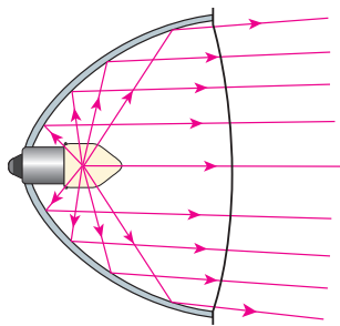
图4.3-7 汽车前灯的反光装置
