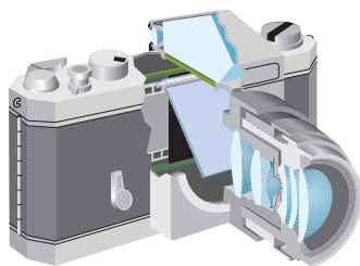
图5.1-1 照相机镜头剖面图
