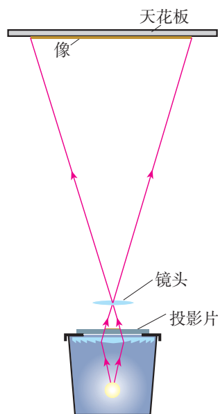
图5.2-4 投影仪成像
