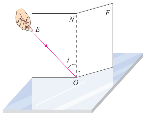
图4.2-4 是否还能看到反射光
