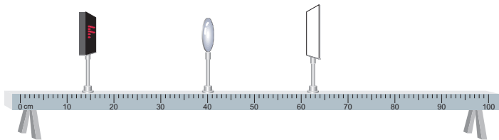
图5.3-2 探究凸透镜成像规律的装置
