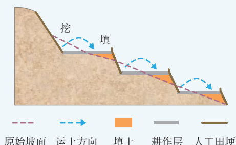
图3.3 修建梯田的主要方式
