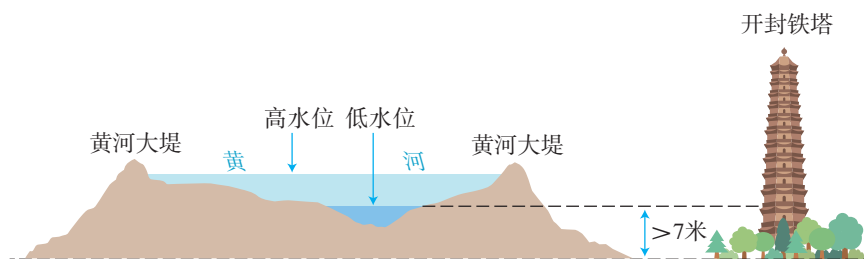
图2.30 开封“地上河”示意
