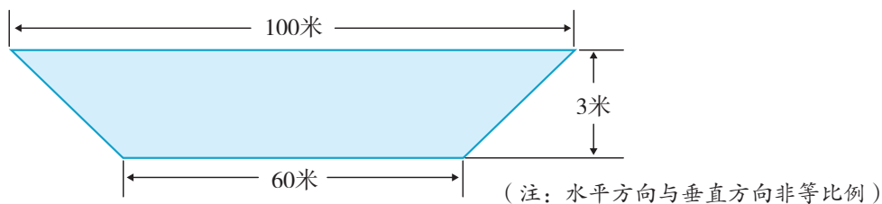
图2.34 河流过水横截面示意
