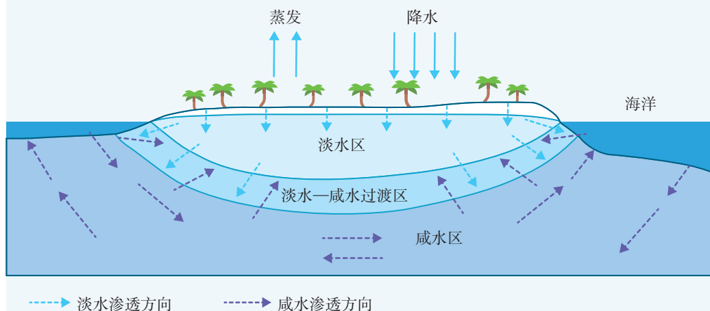
图 3.27 人工岛淡水区形成示意
