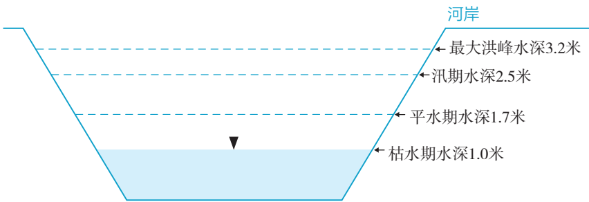
图 2.35 不同水位下的河流横截面示意
