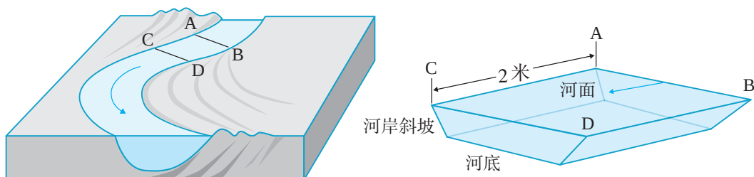
图 2.36 河流某河段流量计算原理示意
