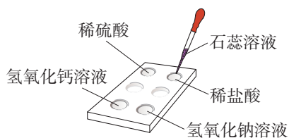
图 10-22 酸、碱与指示剂作用
