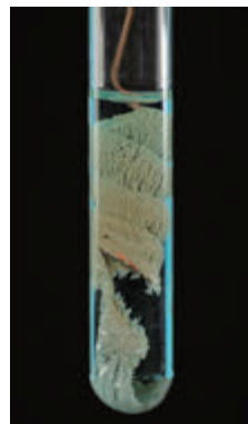
图8-12 铜与硝酸银溶液的反应
