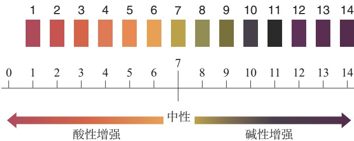
图 10-3 \text{pH} 和溶液的酸碱性
