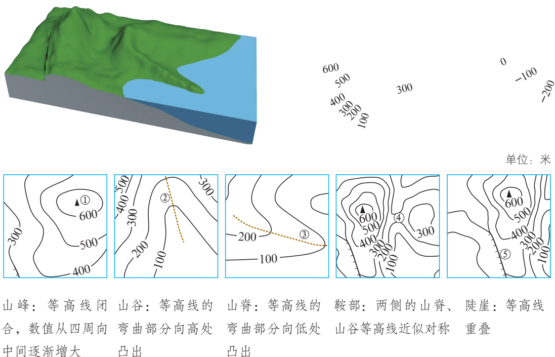
图2.10 等高线地形图上不同的地形部位
