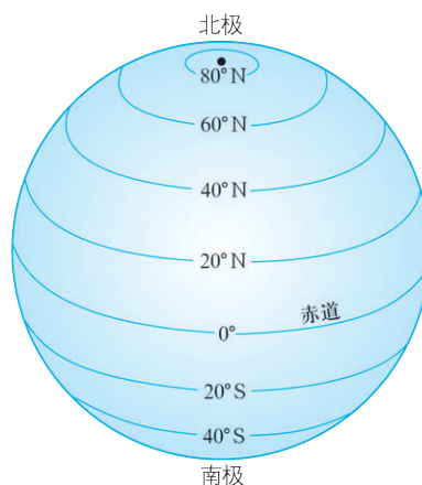
图1.15 纬线和纬度
