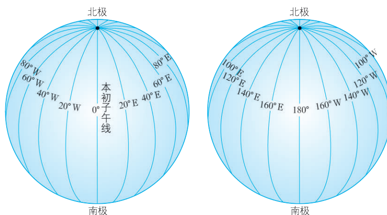
图1.11 经线和经度
