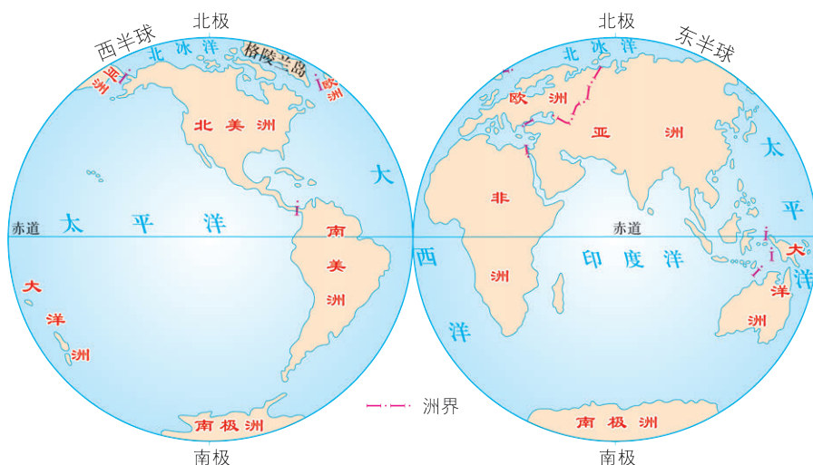
图3.5 大洲的分布
