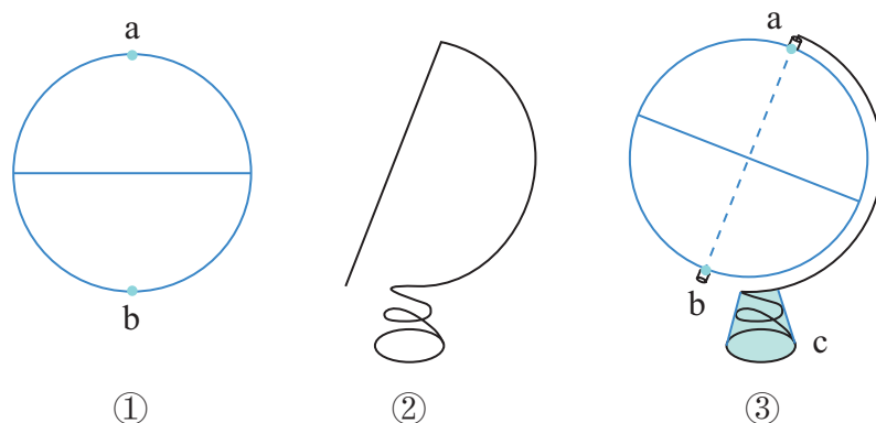
图1.10 制作简易地球仪示意
