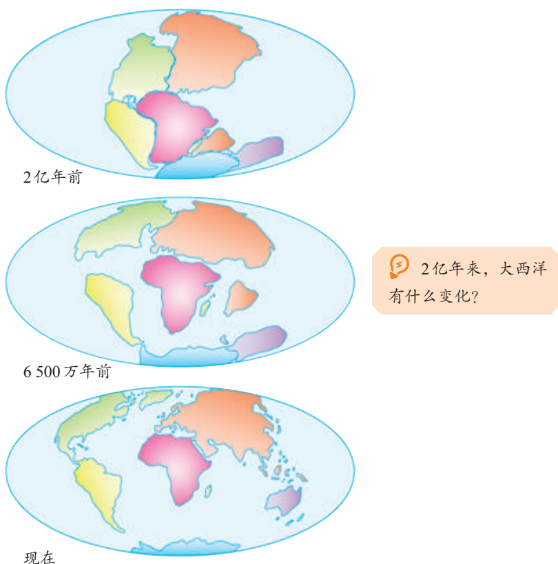
图3.23 大陆漂移
