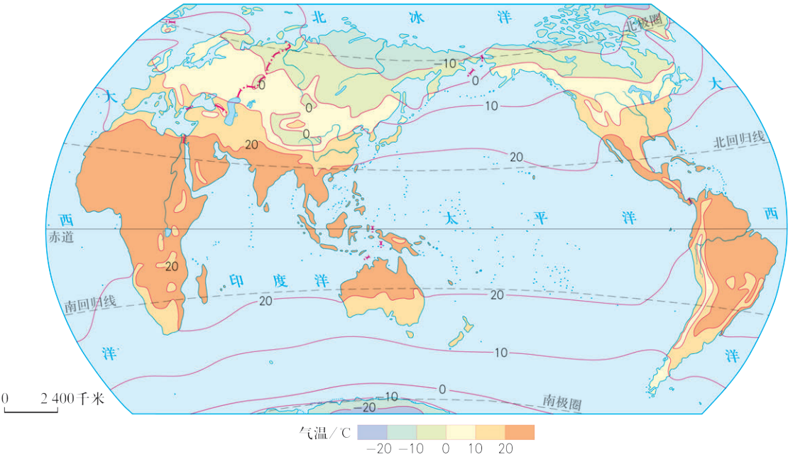
图4.13 世界年平均气温的分布
