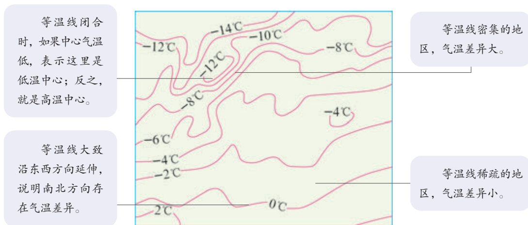
图4.12 等温线的判读方法
