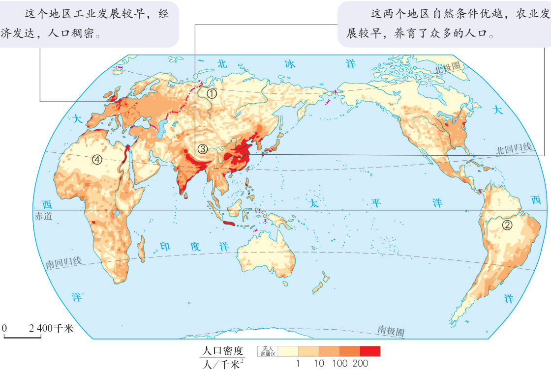
图 5.5 世界人口分布（2017 年）
