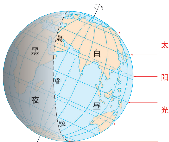
图1.18 昼与夜
