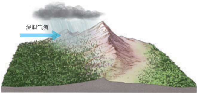
在山地和丘陵地区，海拔每升高 100 米，气温约下降 0.6℃。
